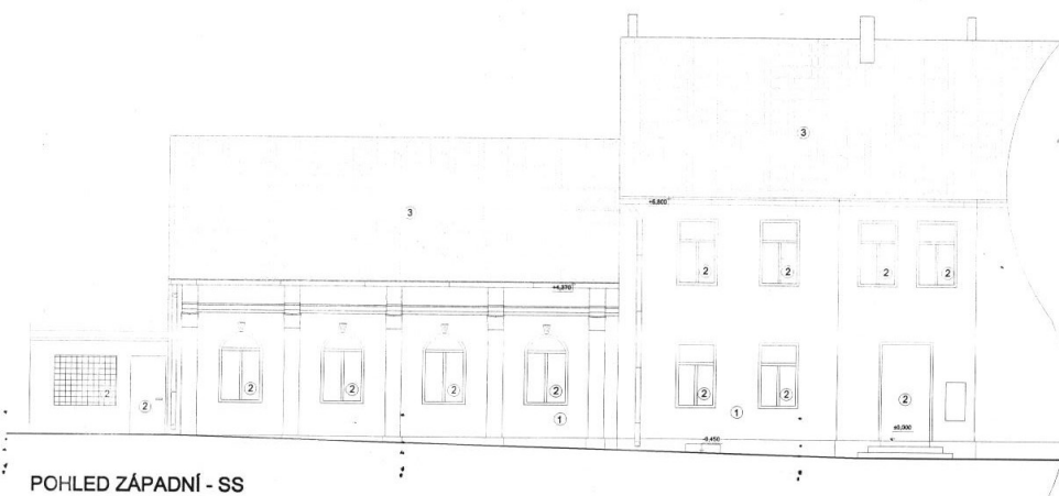
POHLED ZÁPADNÍ - SS
